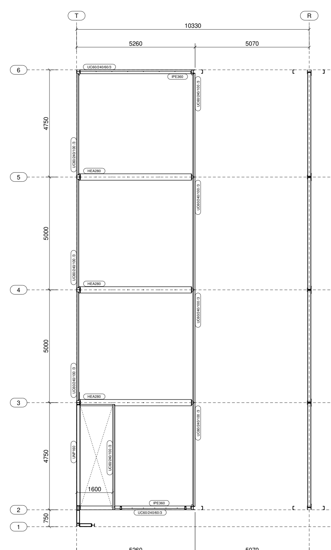
Verdieping
